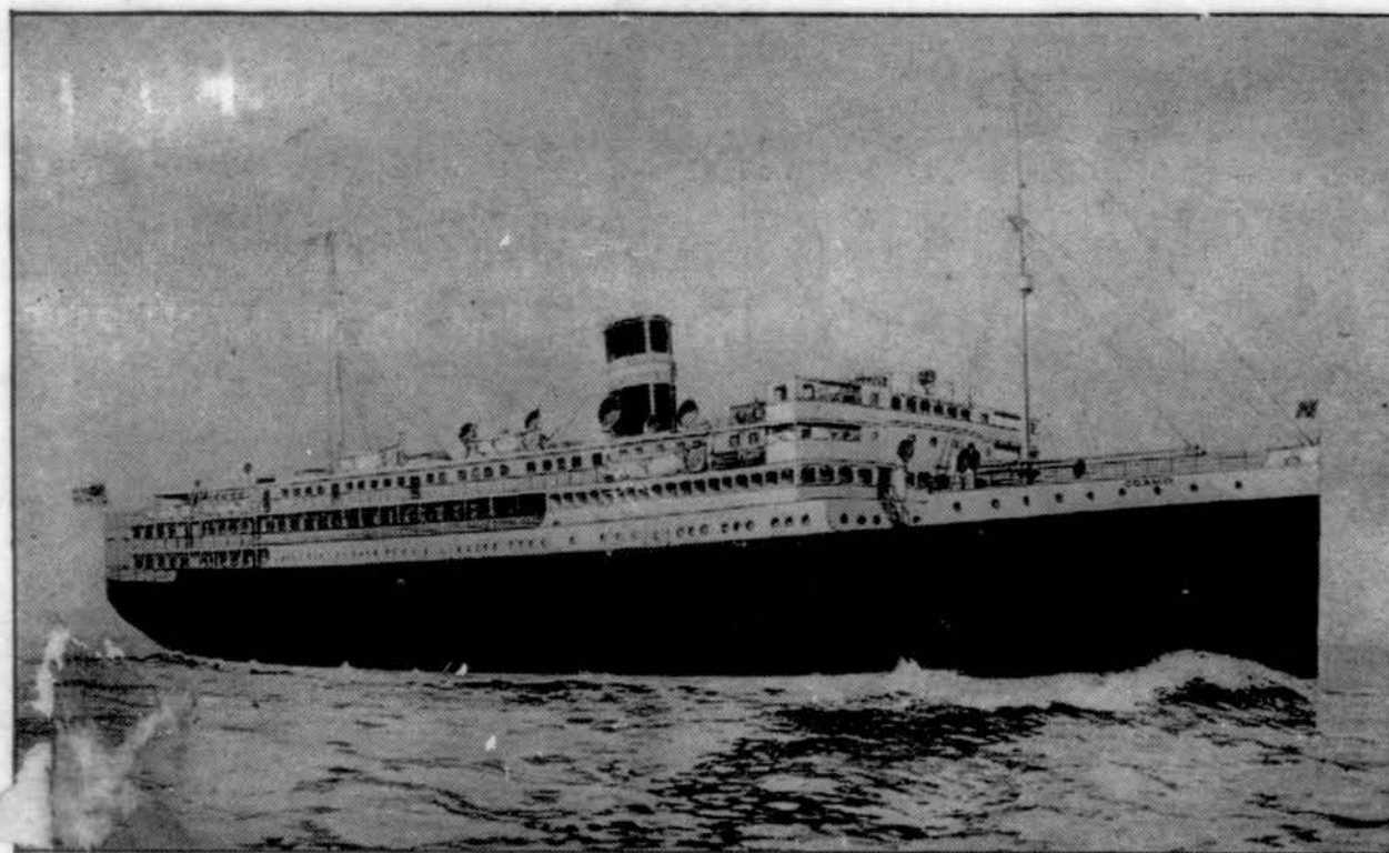
VAPOR "BORINQUEN"
